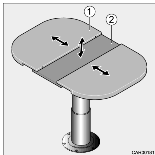
Slika 75 Raztezanje mizne plošče
