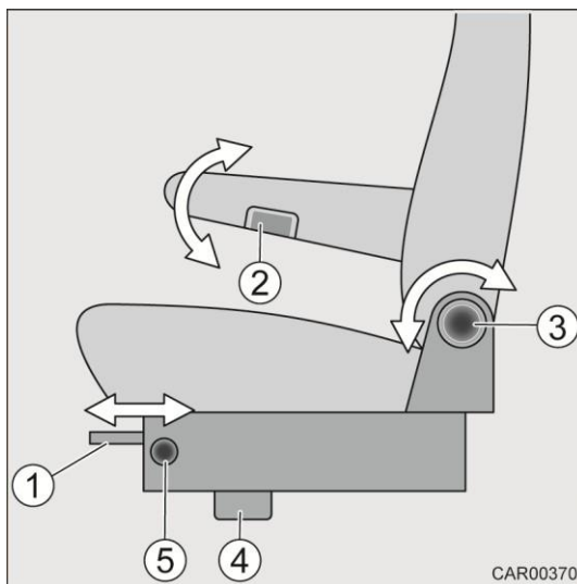
Slika 23 Sedež z nastavitvijo višine in naklona
