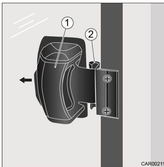
Slika 60 Zaklepni mehanizem
