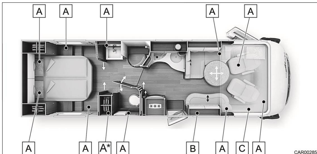
Slika 185 Položaji namestitve pri različici z zakonsko posteljo in XL kopalnico
