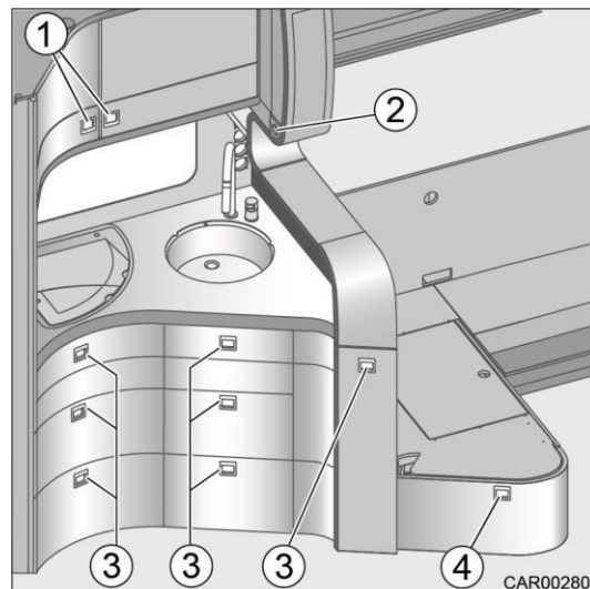
Slika 109 Centralno zaklepanje za kuhinjske elemente in predal za čevlje
