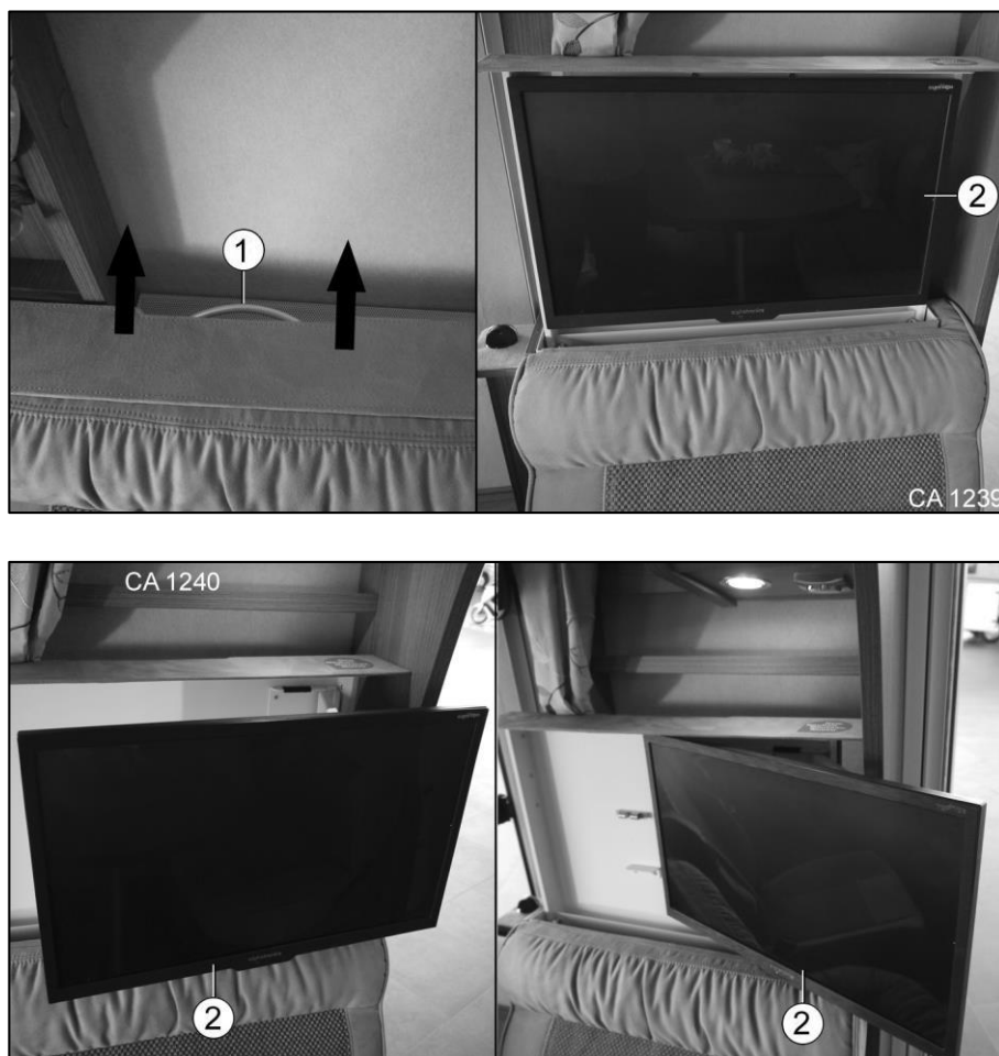
Slika 152 Izvlečni TV nosilec TFT na stranski sedežni klopi
