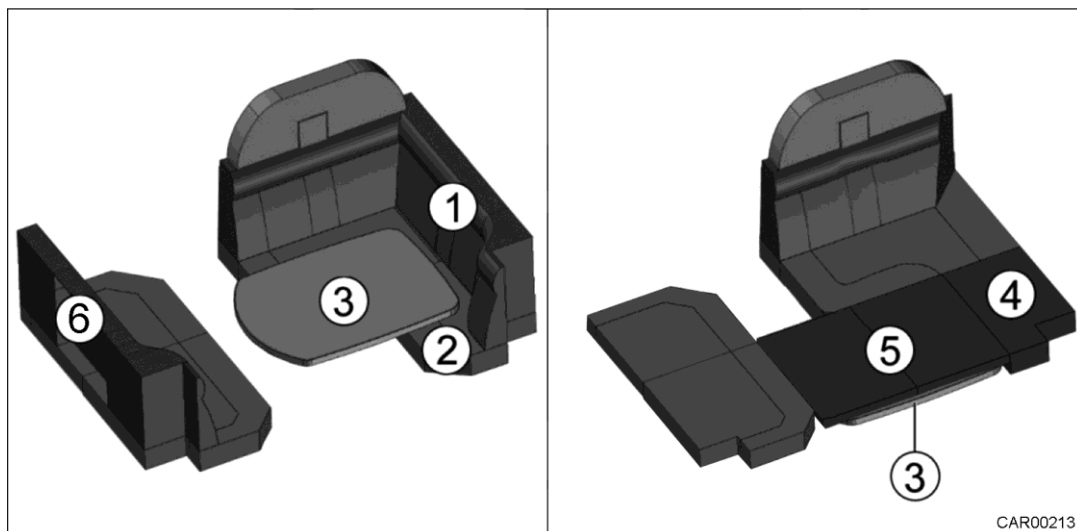
Slika 79 Preureditev sedežne skupine v ležišče
