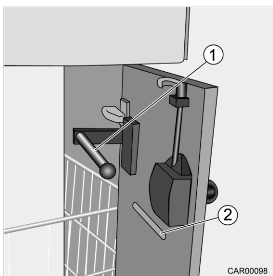
Slika 178 Držalo za toaletni papir na vratih elementa
