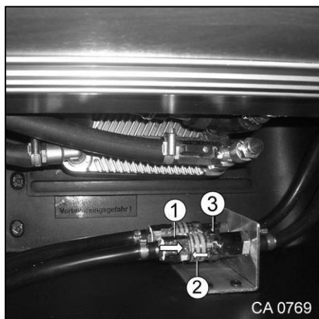
Slika 141 Priključki za talno ogrevano podlogo v voznikovi kabini
