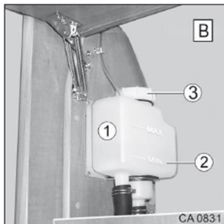
Slika 188 Ekspanzijska posoda
