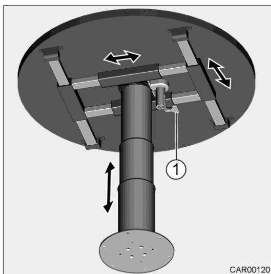
Slika 76 Spuščanje (brez ročice) in premikanje (z ročico) mize
