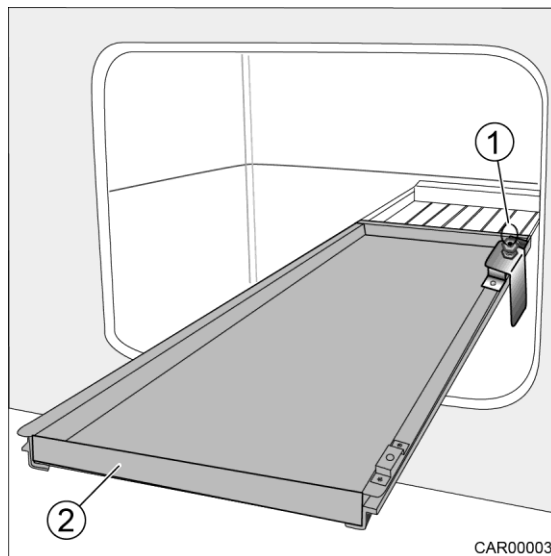
Slika 2 Izvelčni sistem
