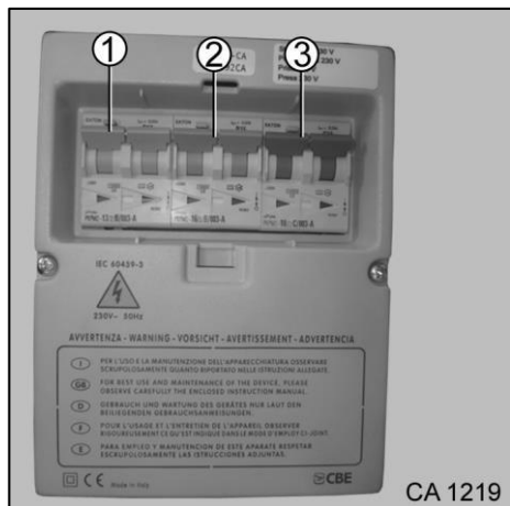
Slika 118 Tokovna zaščitna stikala FID
