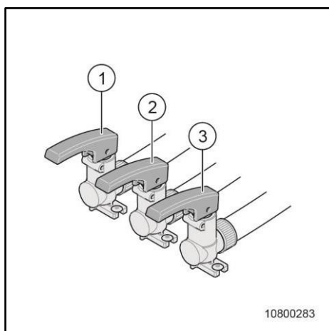
Slika 159 Izpustne pipe za zmanjšanje teže, boiler in svežo vodo
