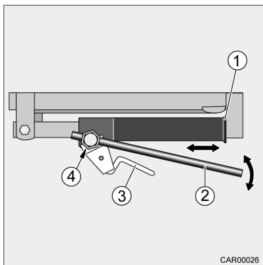
Slika 43 Podporne noge pri modelu s-plus
