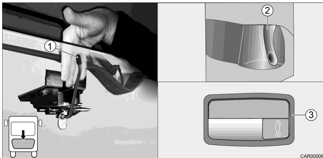
Slika 12 Odpiranje pokrova motorja
