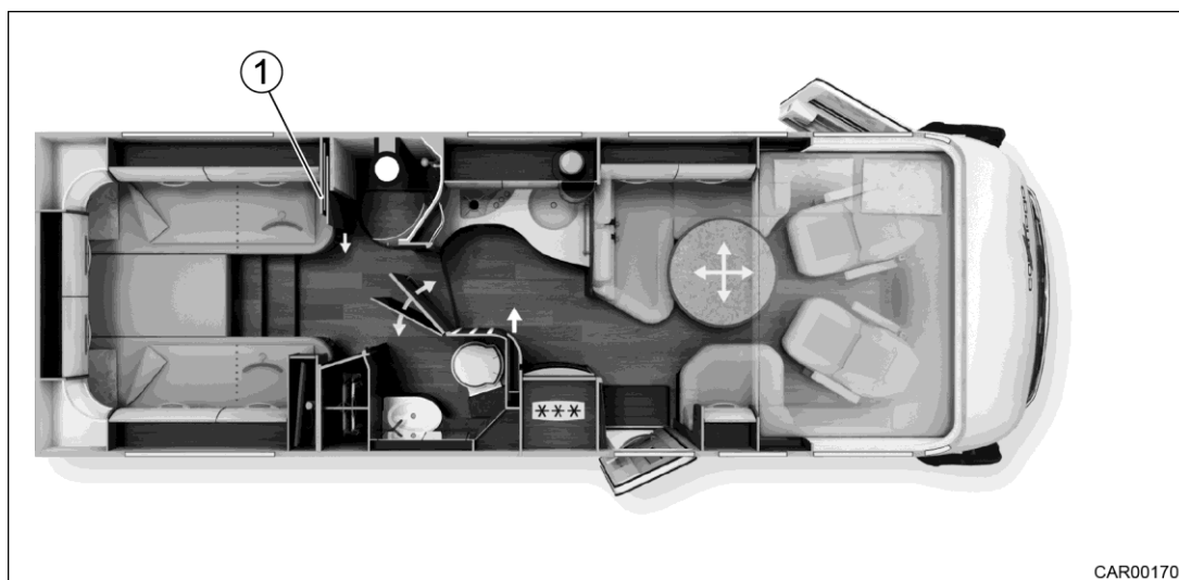
Slika 99 Prestižna kopalnica z garderobo (dvojna vrata) in vzdolžnim enojnim ležiščem
