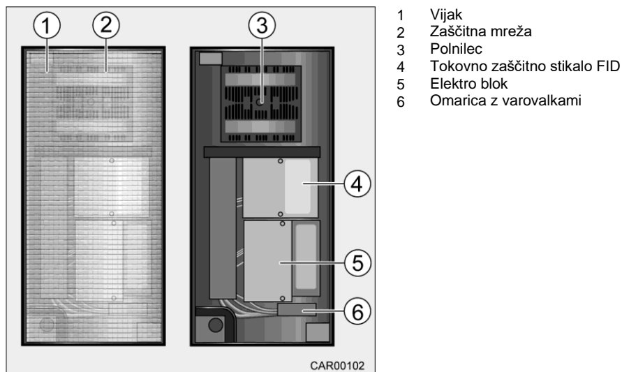
Slika 124 Elektro blok v zadnji garaži
