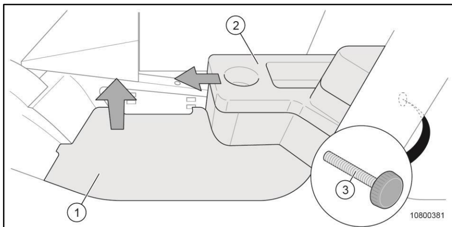
Slika 209 Zamenjava zagonskega akumulatorja
