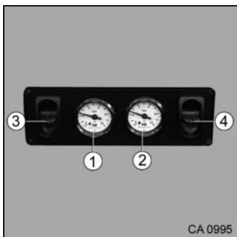
Slika 42 Merilnik tlaka komprimiranega zraka za dodatno pnevmatsko vzmetenje
