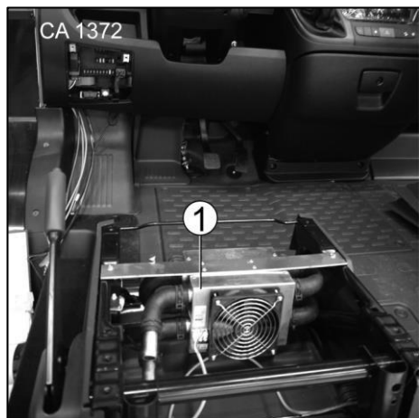
Slika 142 Pospeševalnik gretja
