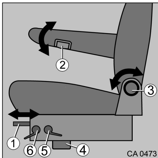
Slika 21 Sedež z nastavitvijo višine in naklona
