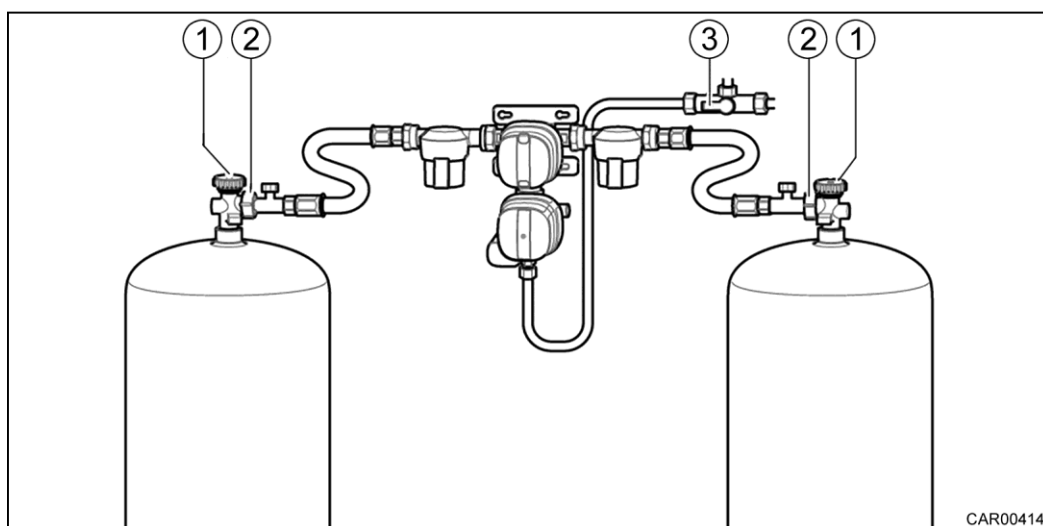
Slika 129 Plinske jeklenke s sistemom za regulacijo plina
