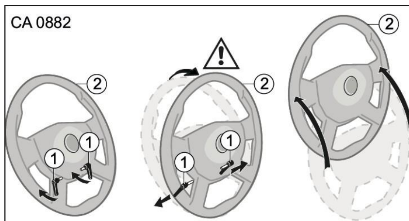
Slika 82 Premik volanskega obroča
