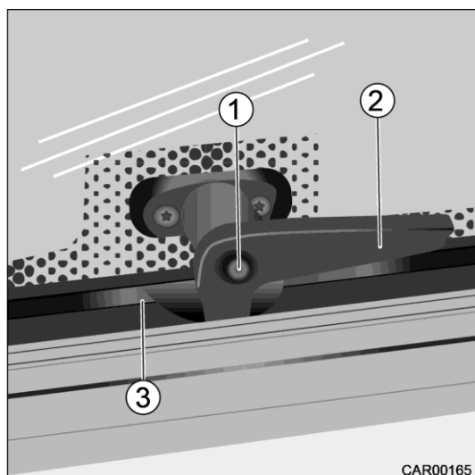
Slika 62 Zaklepni mehanizem nagibnega okna
