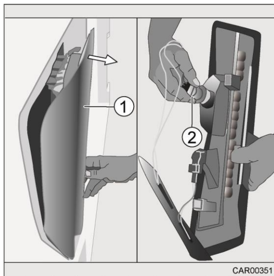
Slika 204 Zamenjava žarnice zadnje luči
