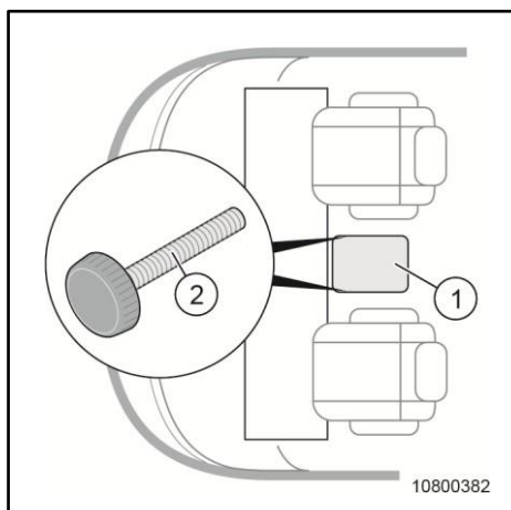
Slika 210 Zamenjava zagonskega akumulatorja
