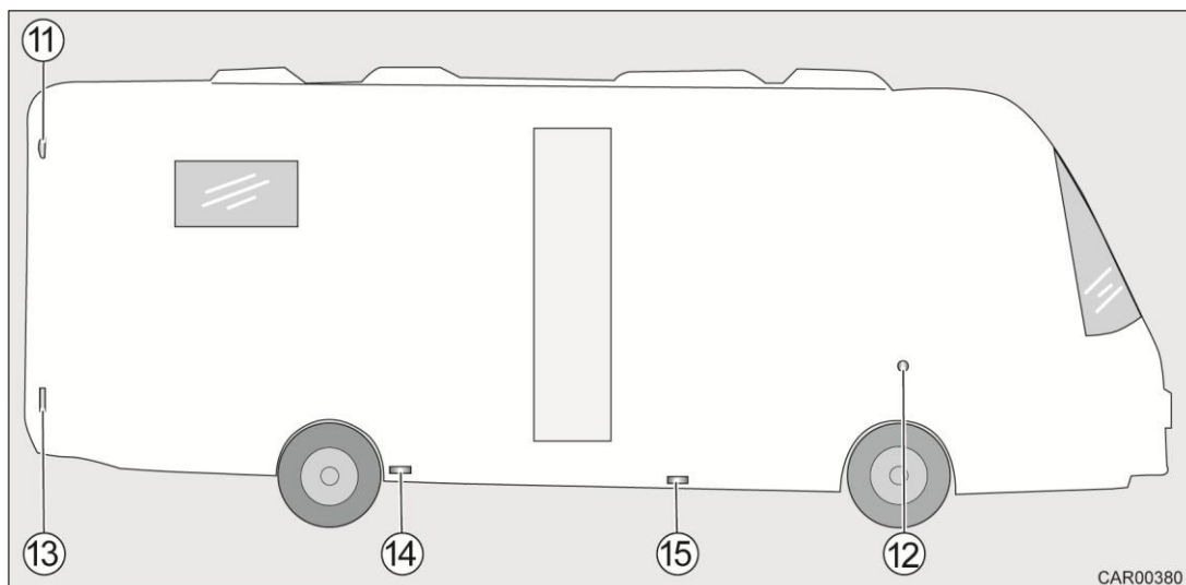
Slika 201 Stranske luči
