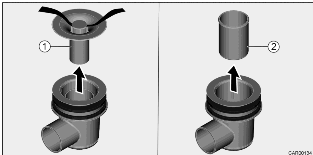
Slika 166 Lovilec neprijetnih vonjav (sifon v tuš kadi), različica s kromiranim pokrovom
