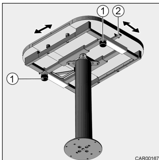
Slika 72 Premikanje mizne plošče
