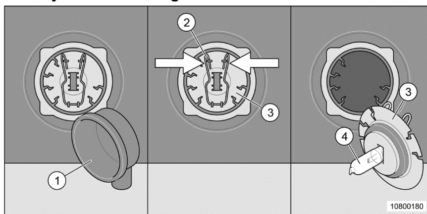
Slika 203 Zamenjava žarnice meglenske / dnevnih luči
