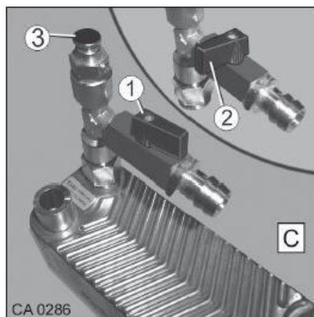
Slika 189 Toplotni izmenjevalnik motorja
