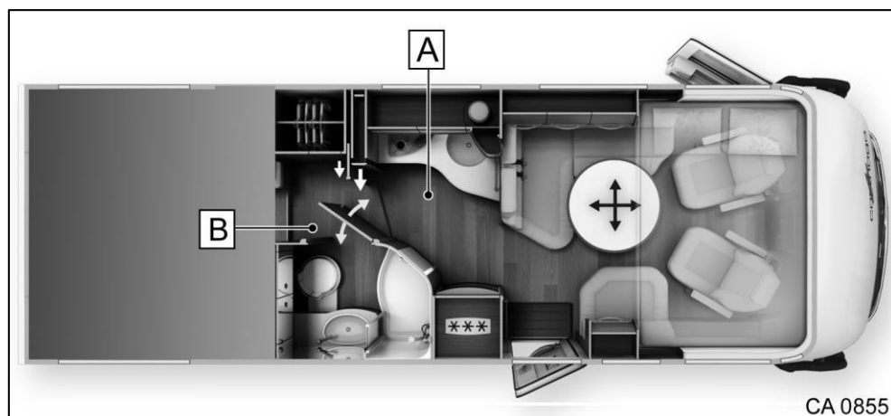
Slika 190 Položaji namestitve senzorjev nivoja vode
