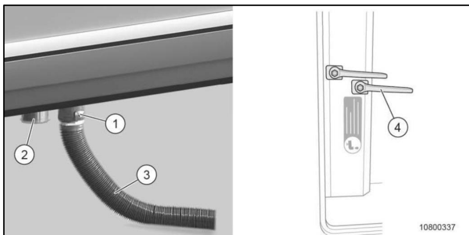
Slika 163 Praznjenje rezervoarja za odpadno vodo
