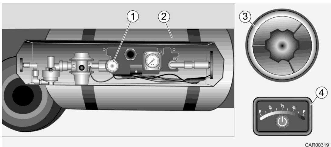
Slika 134 Plinski tank, polnilno grlo tanka in daljinski prikazovalnik količine plina
