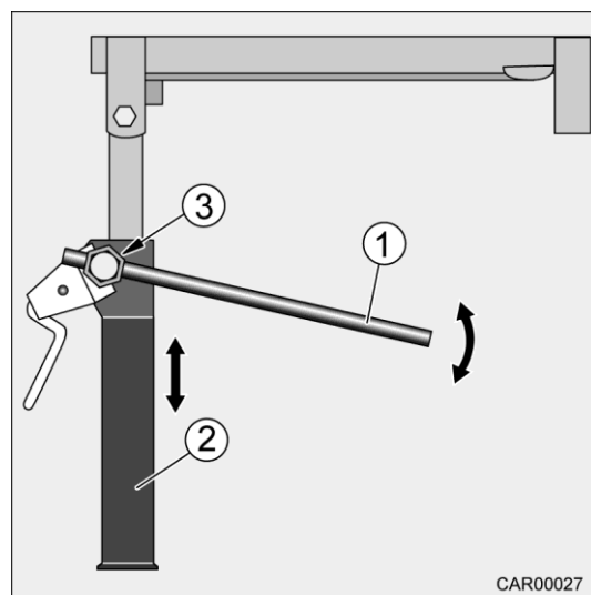
Slika 44 Podporne noge pri modelu s-plus
