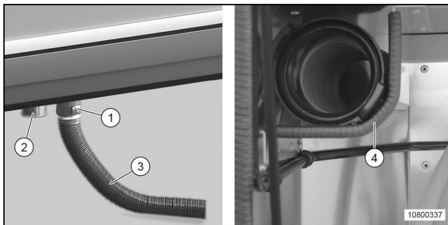
Slika 162 Lokacija izpusta vode/iztočne cevi
