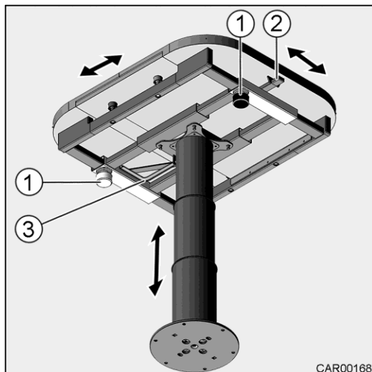
Slika 74 Spuščanje in premikanje mizne plošče
