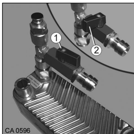
Slika 139 Zapiralni ventil, toplotni izmenjevalnik
