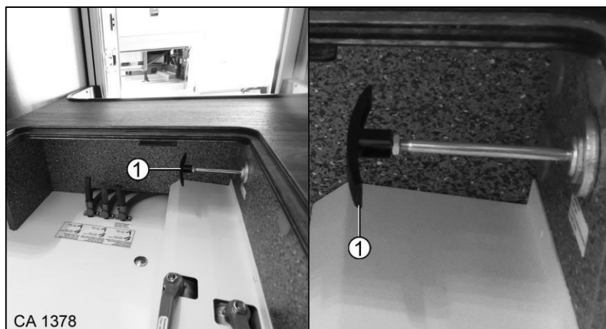
Slika 169 Ročica izpustnega drsnega ventila rezervoarja za fekalije
