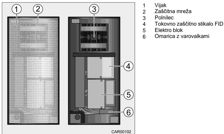
Slika 108 Elektro blok v zadnji garaži
