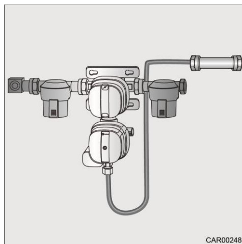
Slika 114 Sistem za regulacijo plina
