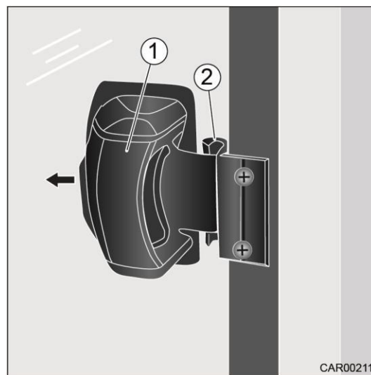
Slika 47 Zaklepni mehanizem
