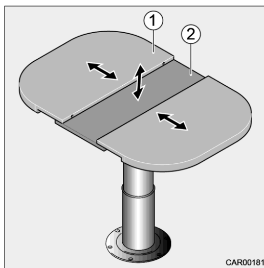
Slika 62 Raztezanje mizne plošče
