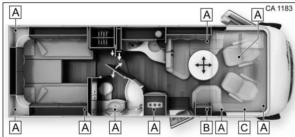
Slika 163 Položaji namestitve pri različici z enojnim ležiščem
