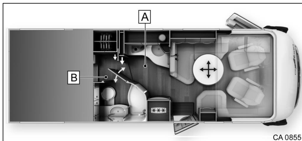
Slika 170 Položaji namestitve senzorjev nivoja vode
