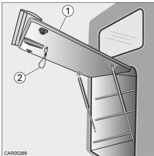
Slika 45 Loputa zadnje garaže, trak za zapiranje lopute
