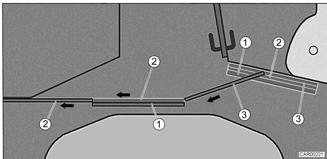
Slika 86 Tloris garderobe (tridelna drsna vrata)
