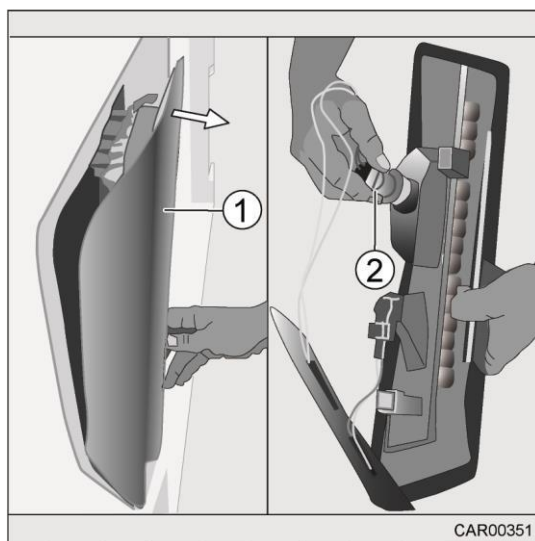
Slika 184 Zamenjava žarnice zadnje luči
