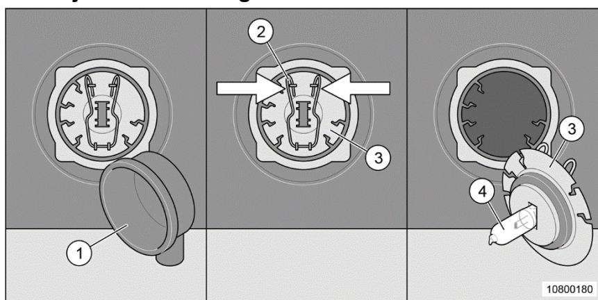
Slika 183 Zamenjava žarnice meglenske / dnevnih luči
