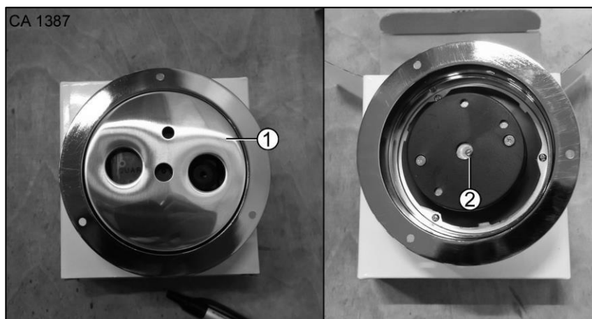
Slika 178 Barometer
