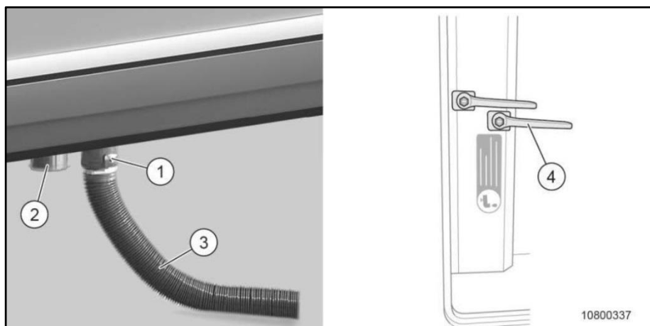
Slika 145 Praznjenje rezervoarja za odpadno vodo
