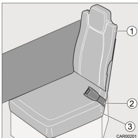
Slika 23 Preureditev stranske sedežne klopi
