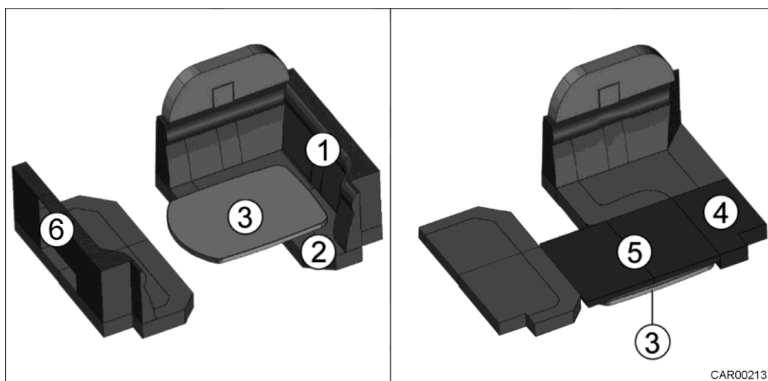
Slika 66 Preureditev sedežne skupine v ležišče
