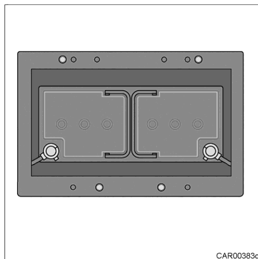
Slika 189 Pokrov zagonskega akumulatorja Slika 190 Zagonski akumulator
