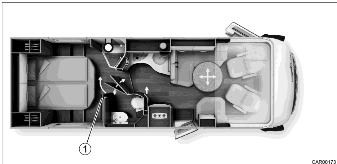
Slika 85 Prestižna kopalnica z garderobo (dvojna vrata in tridelna drsna vrata) in zakonsko posteljo
