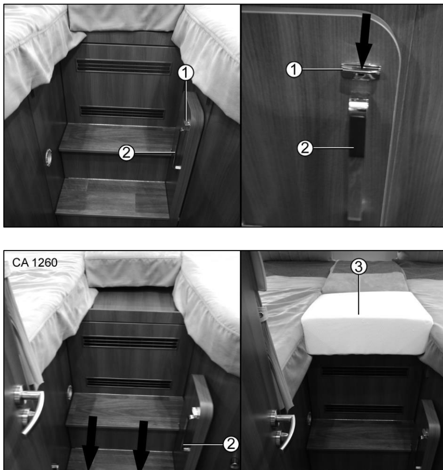
Slika 73 Preureditev ležišča
