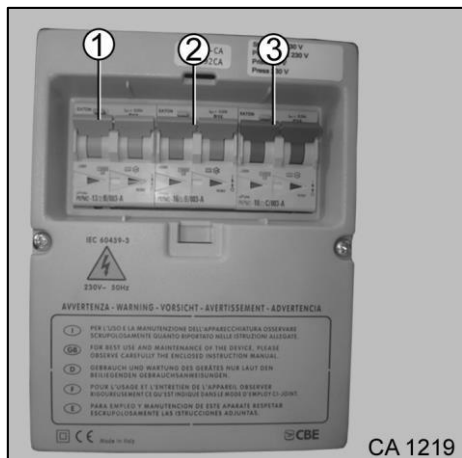
Slika 102 Tokovna zaščitna stikala FID
