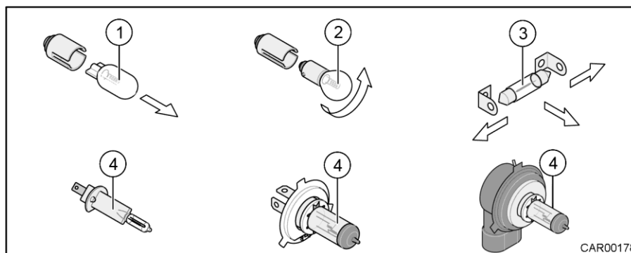
Slika 182 Pregled različnih tipov žarnic
