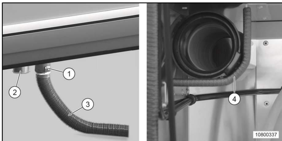
Slika 144 Lokacija izpusta vode/iztočne cevi
