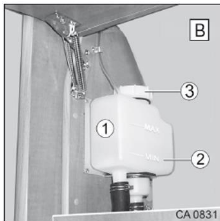
Slika 168 Ekspanzijska posoda
