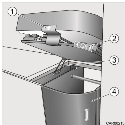
Slika 72 Stransko ležišče
