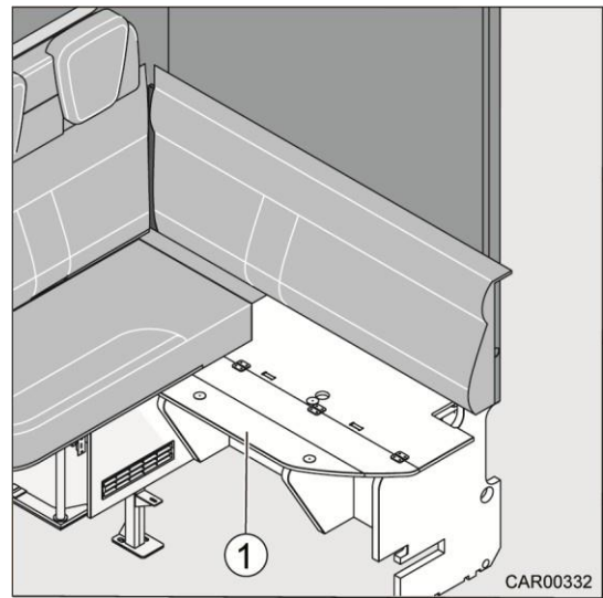
Slika 20 Preureditev vzdolžne sedežne klopi v potovalne sedeže
