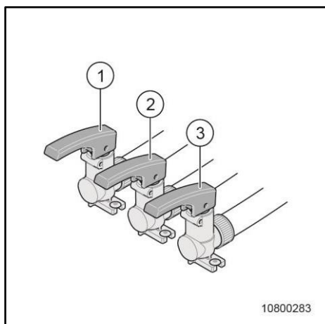
Slika 141 Izpustne pipe za zmanjšanje teže, boiler in svežo vodo
