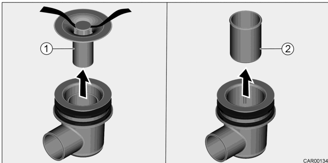
Slika 148 Lovilec neprijetnih vonjav (sifon v tuš kadi), različica s kromiranim pokrovom
