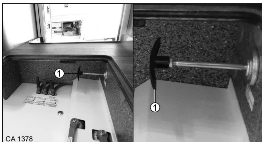
Slika 151 Ročica izpustnega drsnega ventila rezervoarja za fekalije
