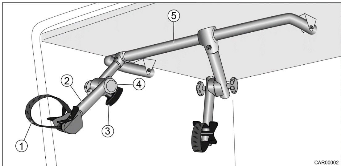
Slika 4 Pritrdilni sistem za električna kolesa v garaži avtodoma
