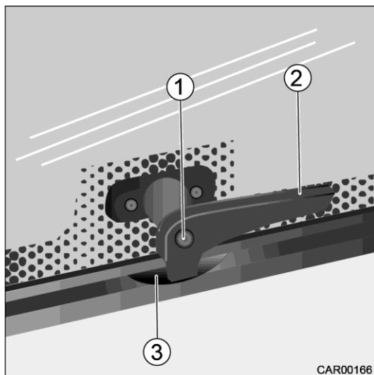
Slika 50 Zaklepni mehanizem nagibnega okna
