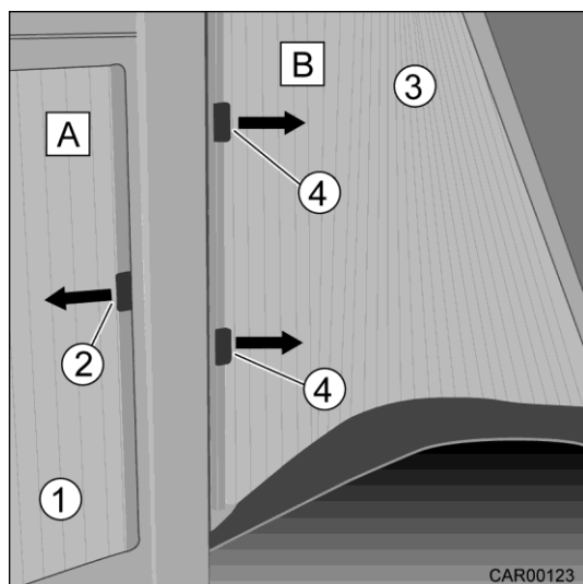
Slika 82 Plise rolo stranskega okna/vrat voznikove kabine
