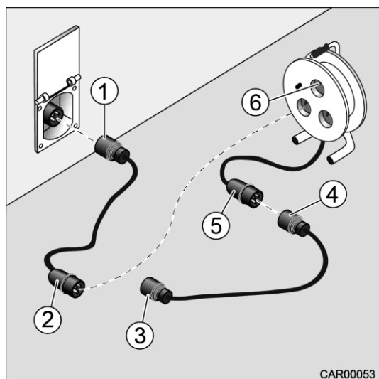
Slika 103 Priključitev kabla
