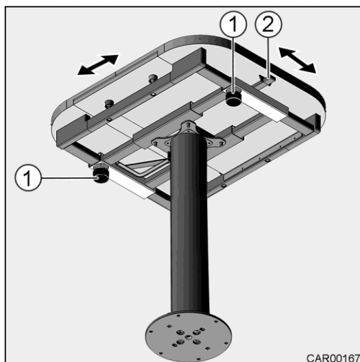
Slika 59 Premikanje mizne plošče
