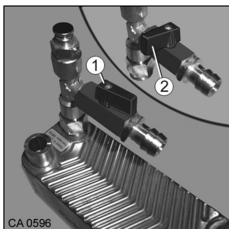
Slika 121 Lokacija zapornega ventila za toplotni izmenjevalnik
