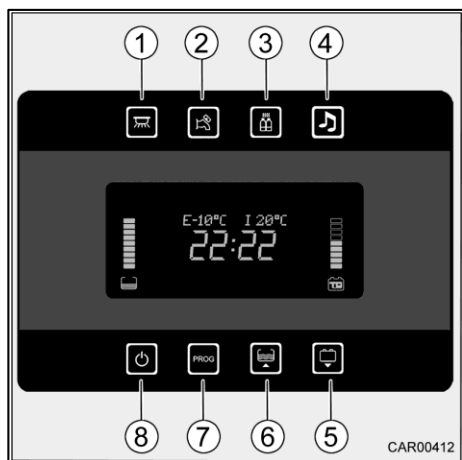
Stikalo 107 Nadzorna plošča
